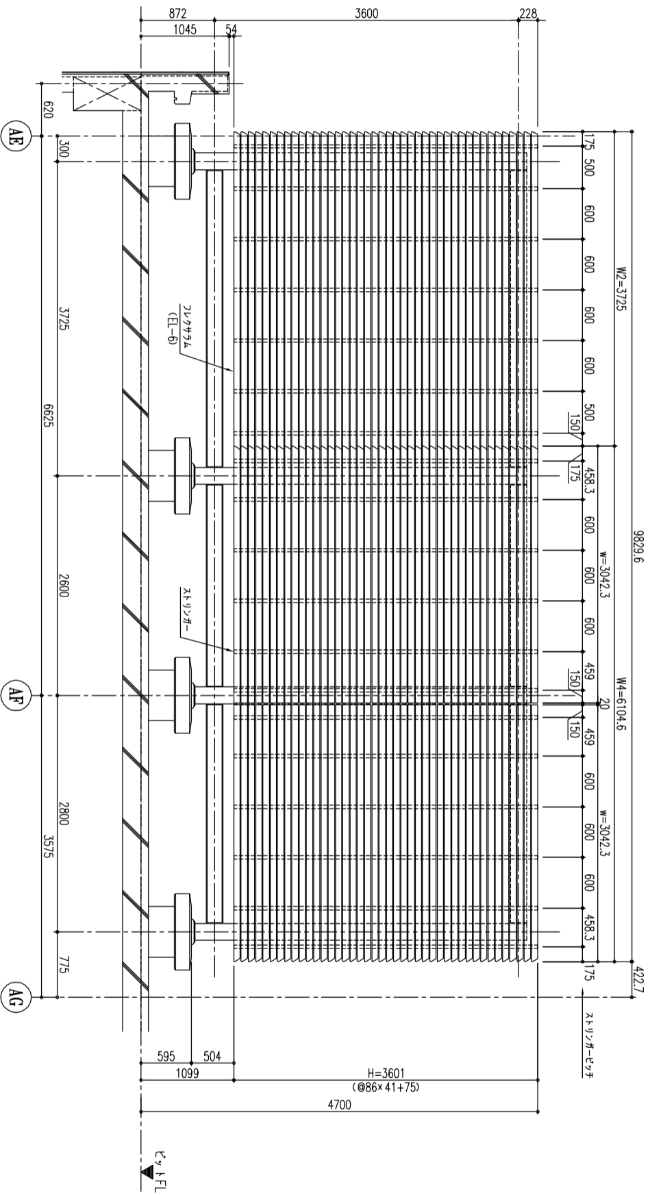
側面 外觀図
