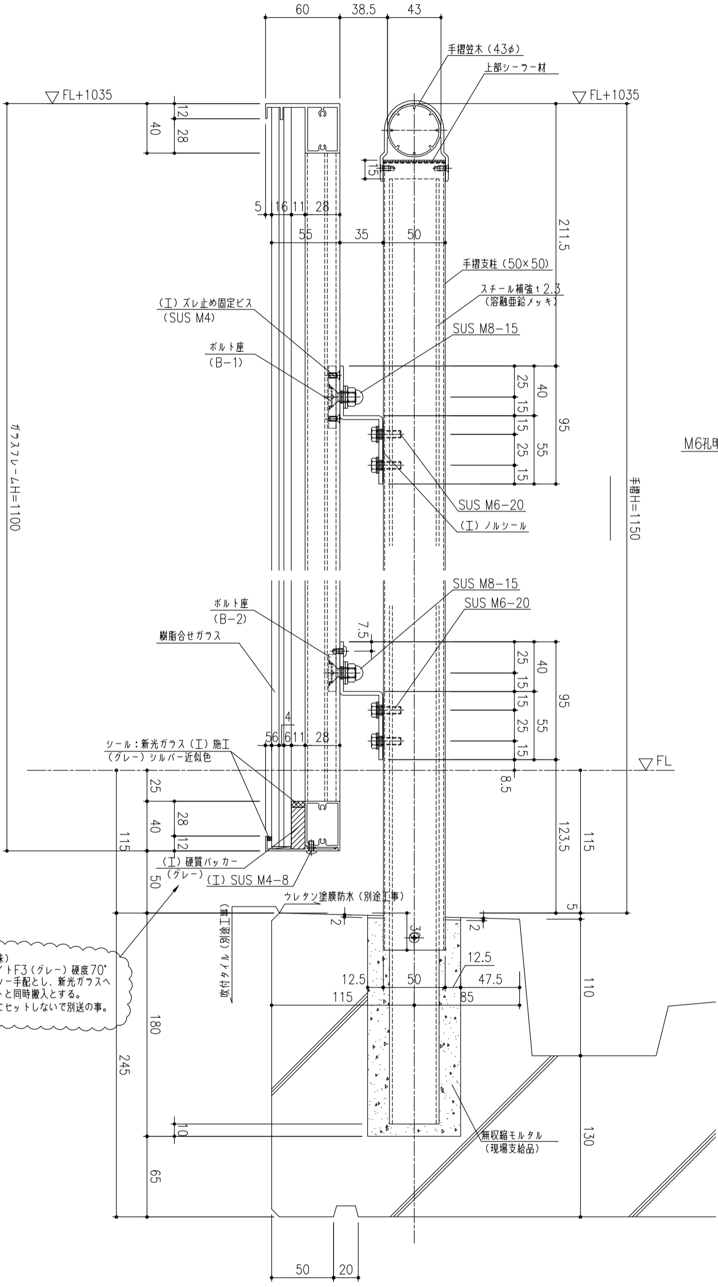
一般部縦断面図
