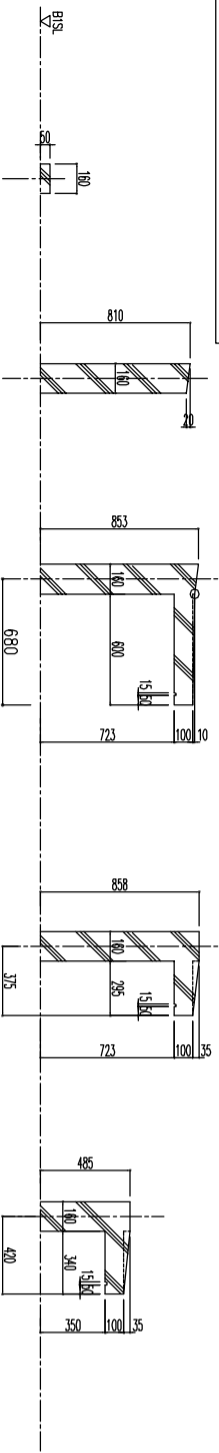
開口部止り部分詳細図 1/20
